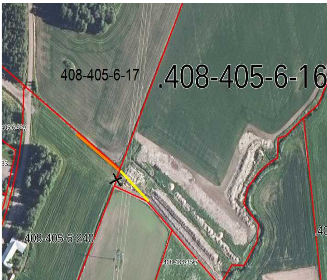
Kuva 1: Oranssilla ja keltaisella ehdotetut salaojat. Musta X ehdotettu vanhan ojan tukkiminen. Pohjoinen rajajoja
